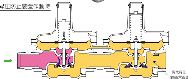
昇圧防止装置作動時
