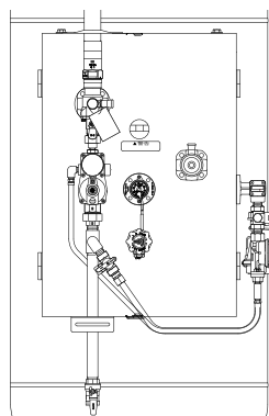
普及型（漏洩検知装置付）
